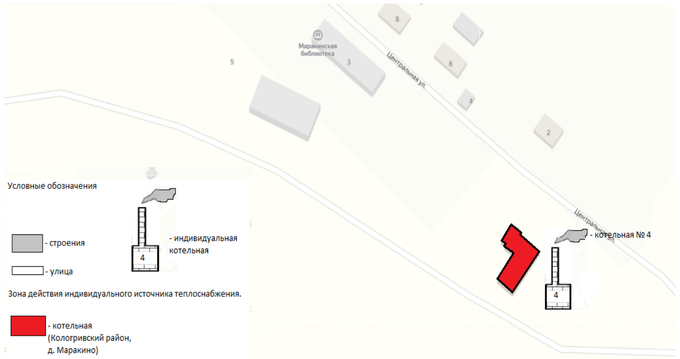
Рисунок 5. Схема индивидуального источника теплоснабжения в д. Марakiно
